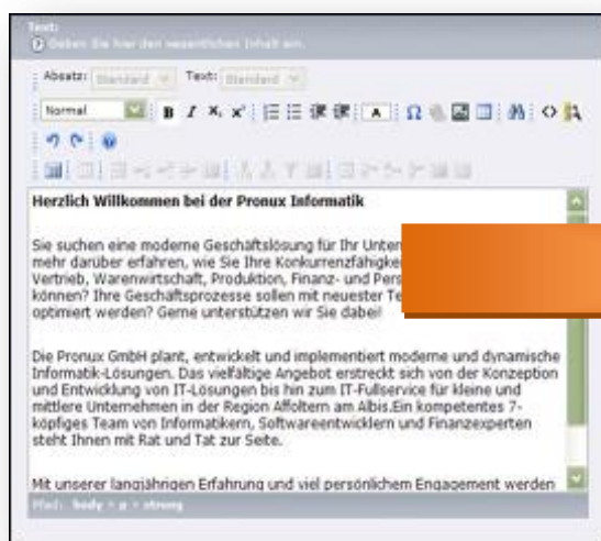
TYPO3 Text-Editor
